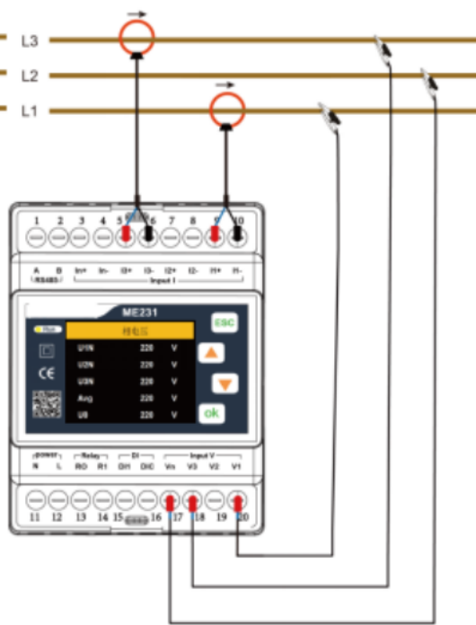
3P3W_2CT
