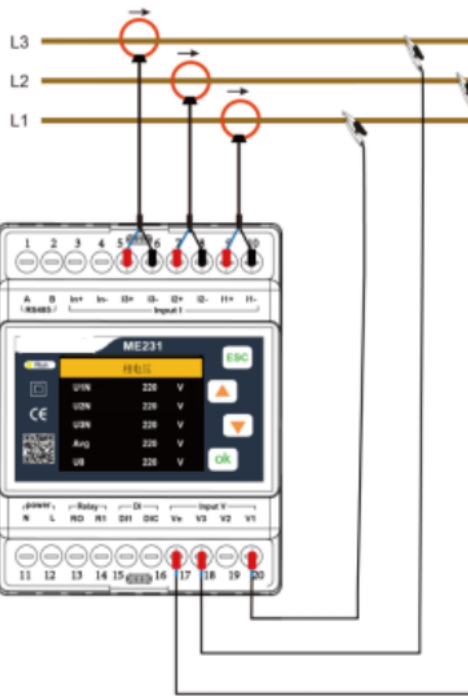
3P3W_3CT
